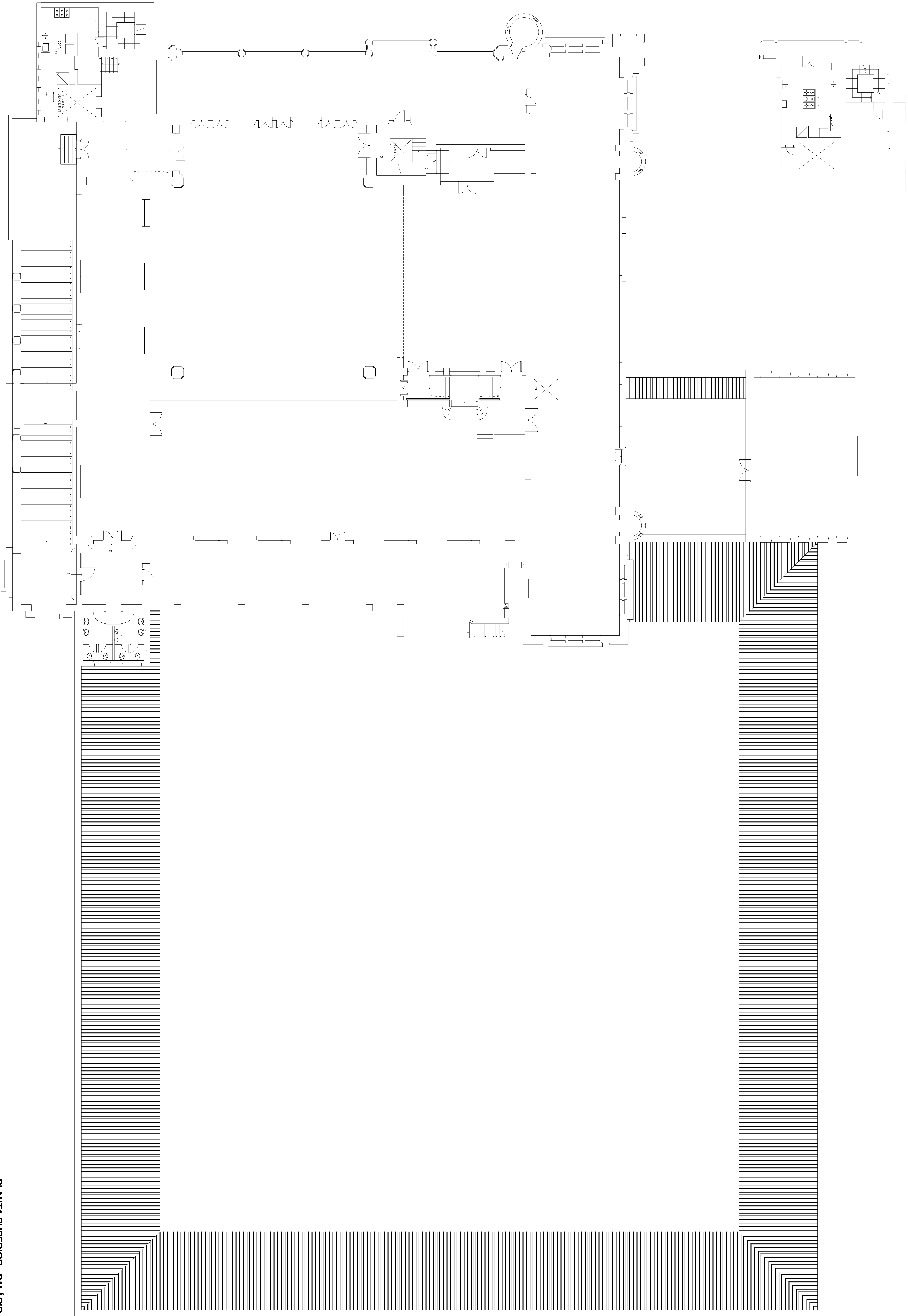
PLANTA SUPERIOR - PALACIO ESC 1:100
